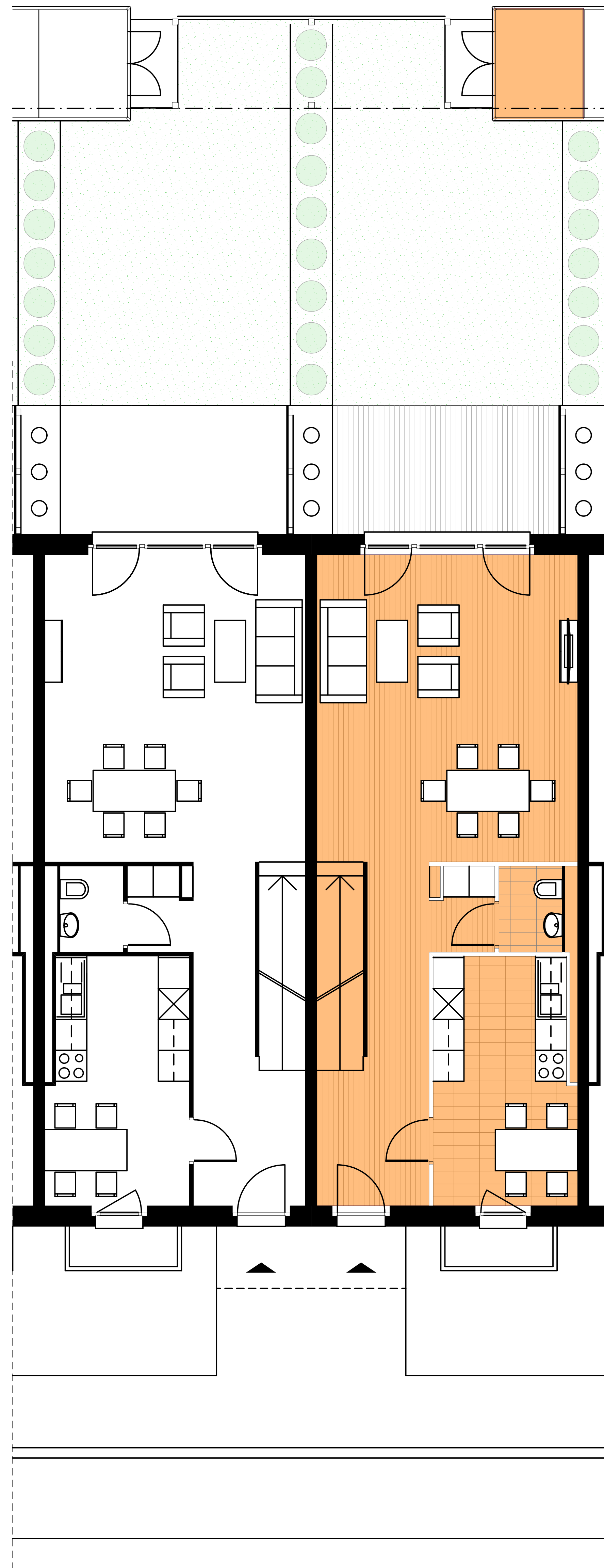
Plan rez-de-chaussée
