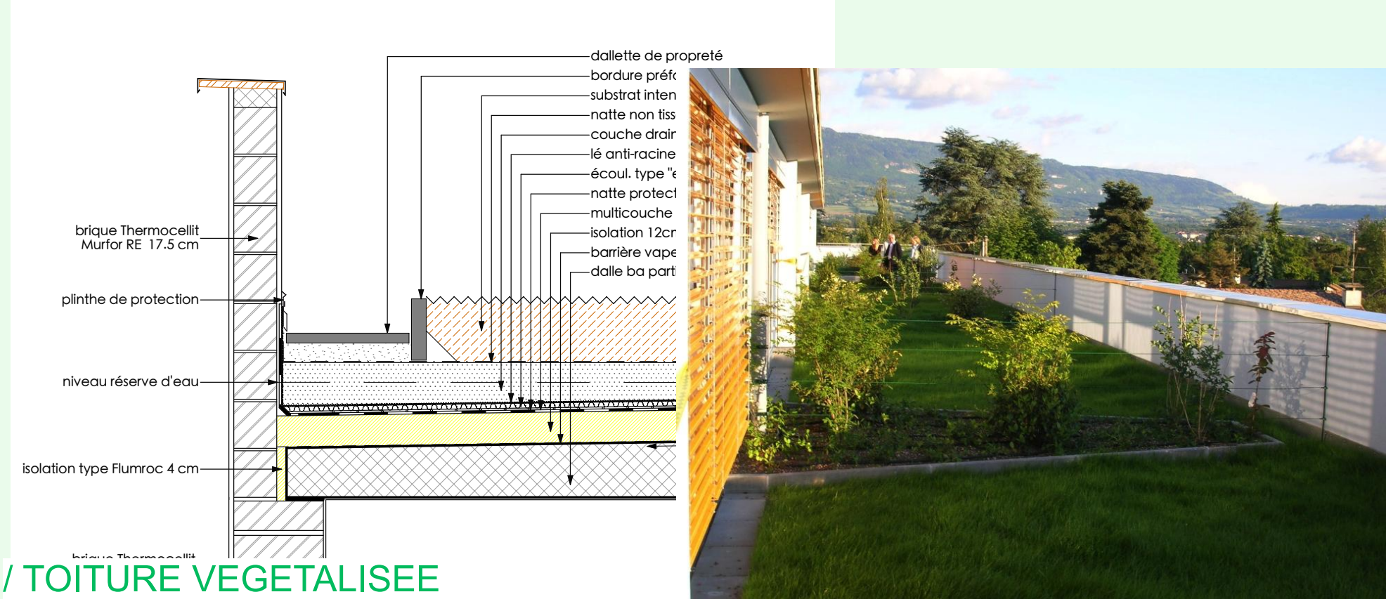
/ TOITURE VEGETALISEE
